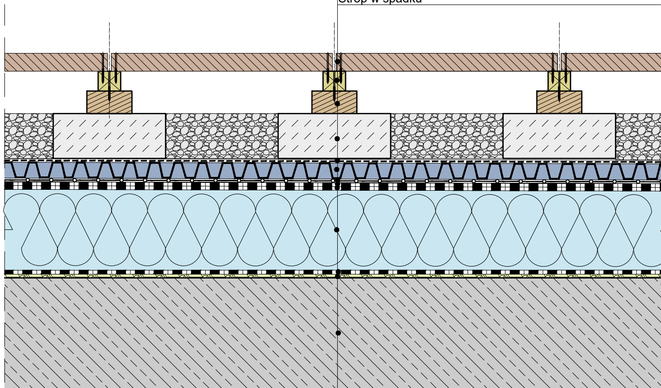
PRZEKRÓJ A-A (WG. DETALU DZ.146)
